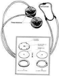
GEOFONO ANALOGO HEATH CONSULTANTS
